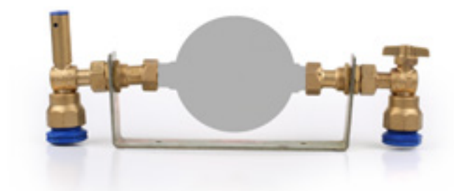
BRANCHEMENT HORIZONTAL AVEC ENTRÉE ÉQUERRE SOPAFLO - SORTIE ÉQUERRE SOPAFLO HORIZONTAL WATER CONNECTING SOLUTION WITH SOPAFLO ELBOW INLET - SOPAFLO ELBOW OUTLET
