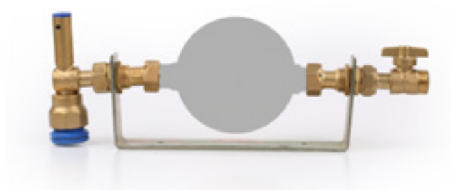
BRANCHEMENT HORIZONTAL AVEC ENTRÉE ÉQUERRE SOPAFLO - SORTIE DROITE SIMPLE HORIZONTAL WATER CONNECTING SOLUTION WITH SOPAFLO ELBOW INLET - SIMPLE STRAIGHT OUTLET
