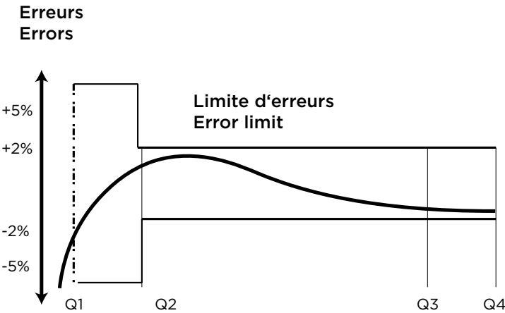
Courbe de précision
