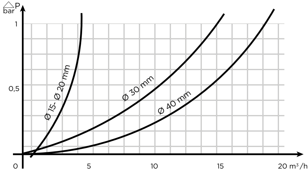
Courbe de perte de charge
