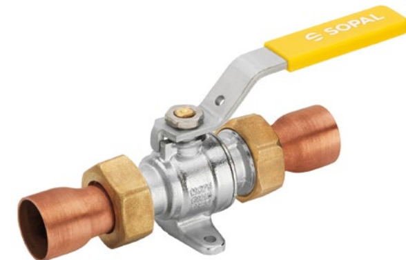
VANNE GAZ A BS APPLIQUE BUSE CUIVRE AVEC LEVIER GAS BALL VALVE WITH FLANGED COUPLING
