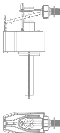
Robinet flotteur coulissant
