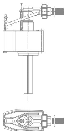
Robinet flotteur coulissant avec embout en laiton
